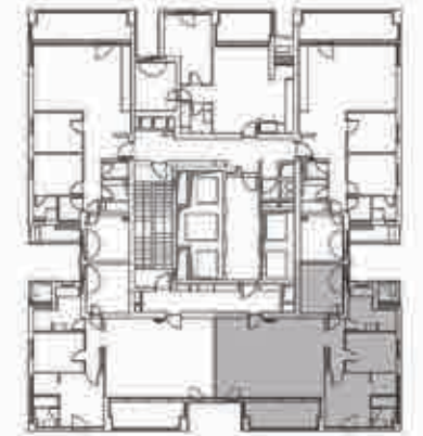
קומות 17 - 42
