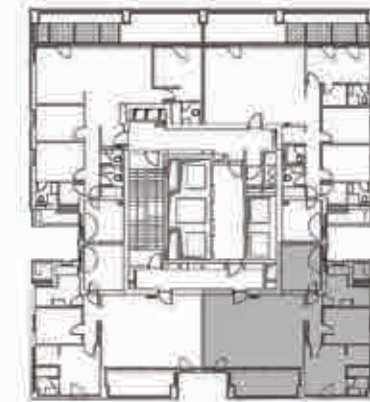
קומה 43
